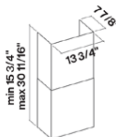
Optional Chimney
