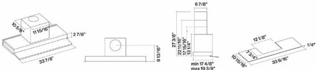
Optional Chimney
